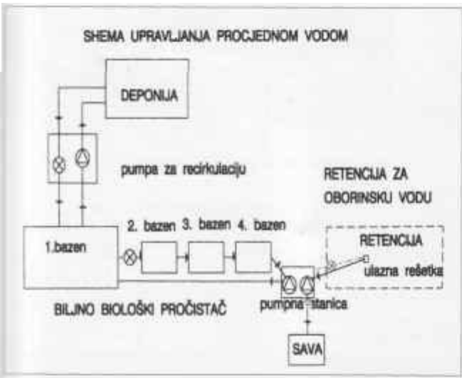
Slika 2: Shematski prikaz biljno-biološkog uređaja za pročišćavanje procjernih voda
